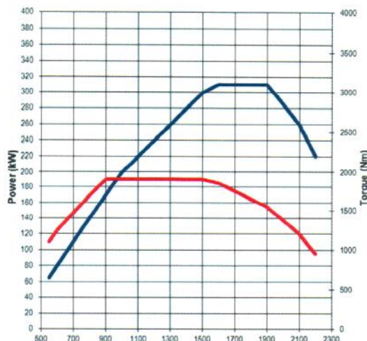
Cursor 13 - 420 HP
