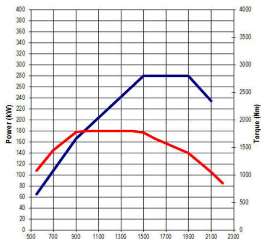
Cursor 13 - 380 HP
